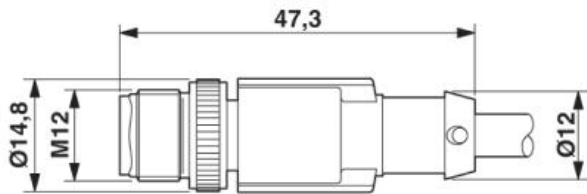
Maßzeichnung, M12 Stecker
