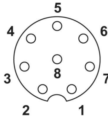
Schaltplan
