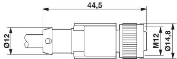
Maßzeichnung, M12 Buchse
