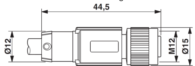
Maßzeichnung
