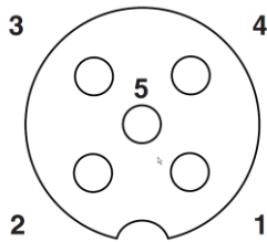
Polbild M12-Buchse, 5-polig, A-kodiert
