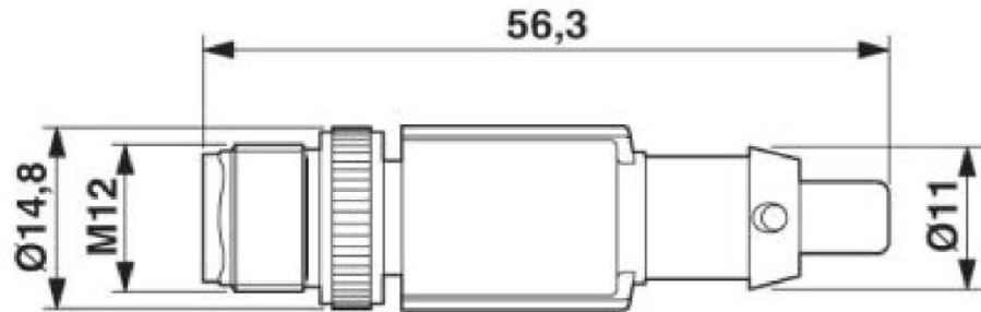
Stecker M12x1, gerade, geschirmt
