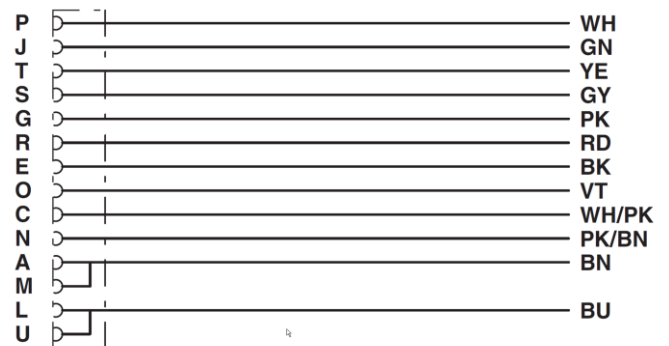
Kontaktbelegung der M16-Buchse
