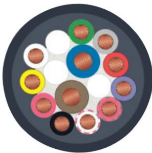
Kabelquerschnitt
