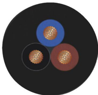
Leitung
