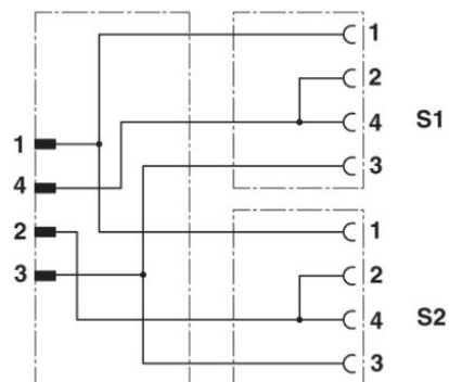
Schaltplan
