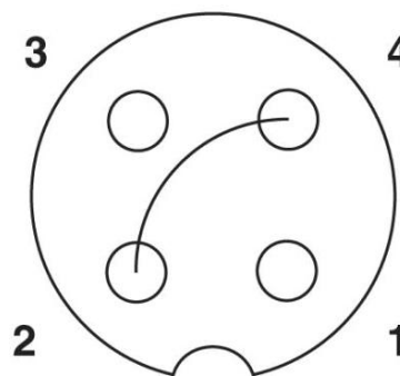
Schaltplan
