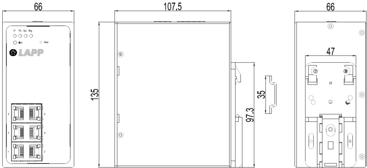
Maßzeichnung (M06T-2GEN)
