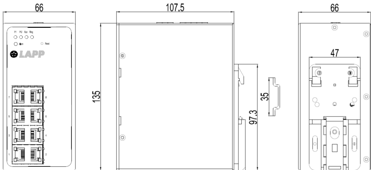
Maßzeichnung (M08T-2GEN)
